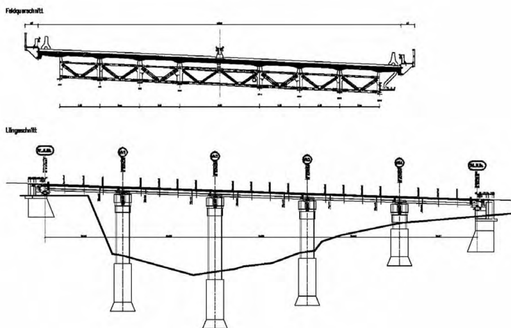
Querschnitt und Längsschnitt nach Brückenumbau und Instandsetzung.
