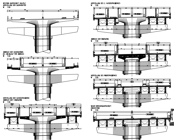
Bauablauf Bauphasen mit Verkehrsführung
